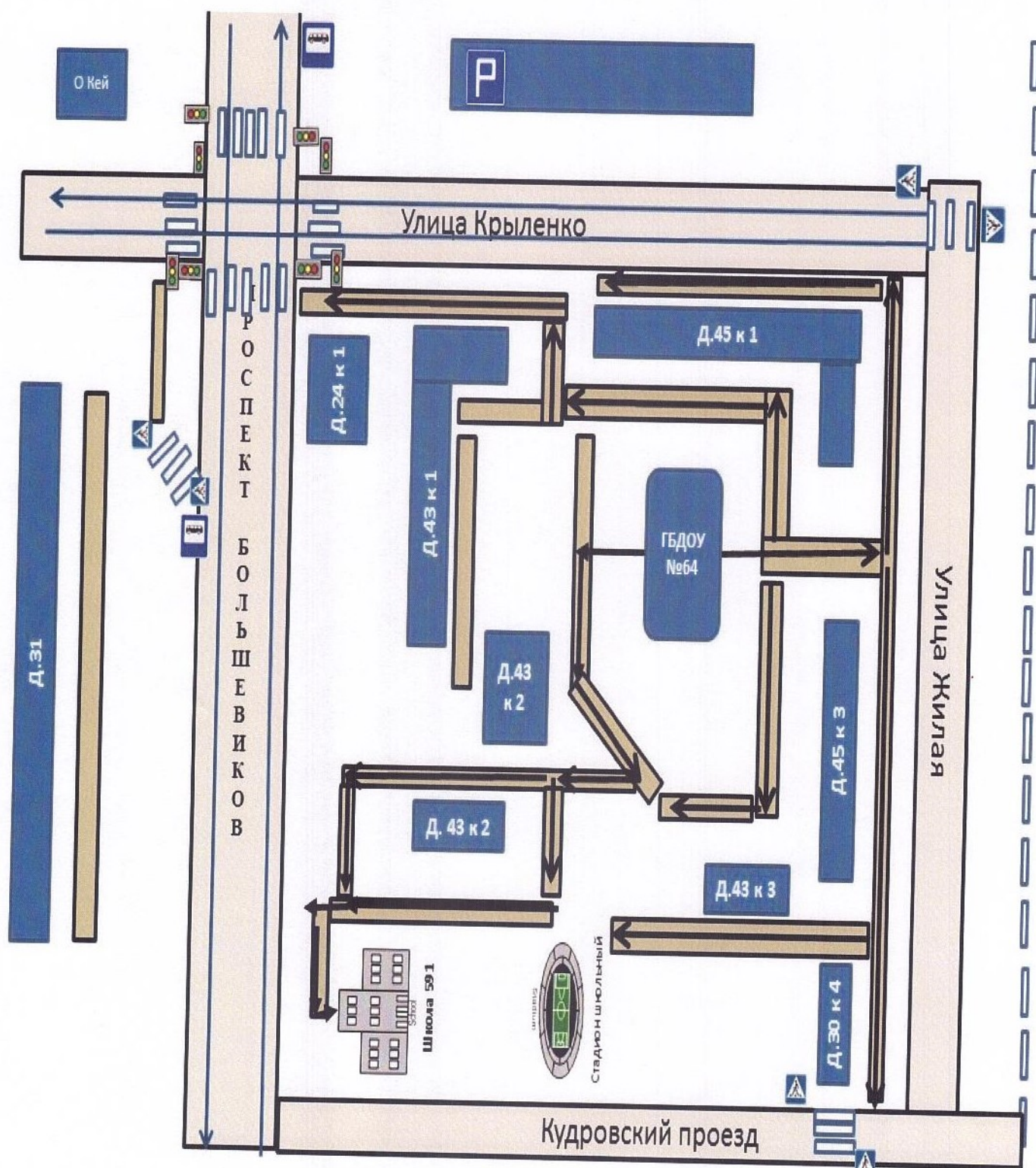
2. Схема организации дорожного движения в непосредственной близости от ГБДОУ детского сада № 64 комбинированного вида неевского района Санкт-Петербурга с размещением соответствующих технических средств, маршруты движения детей и расположение парковочных мест
